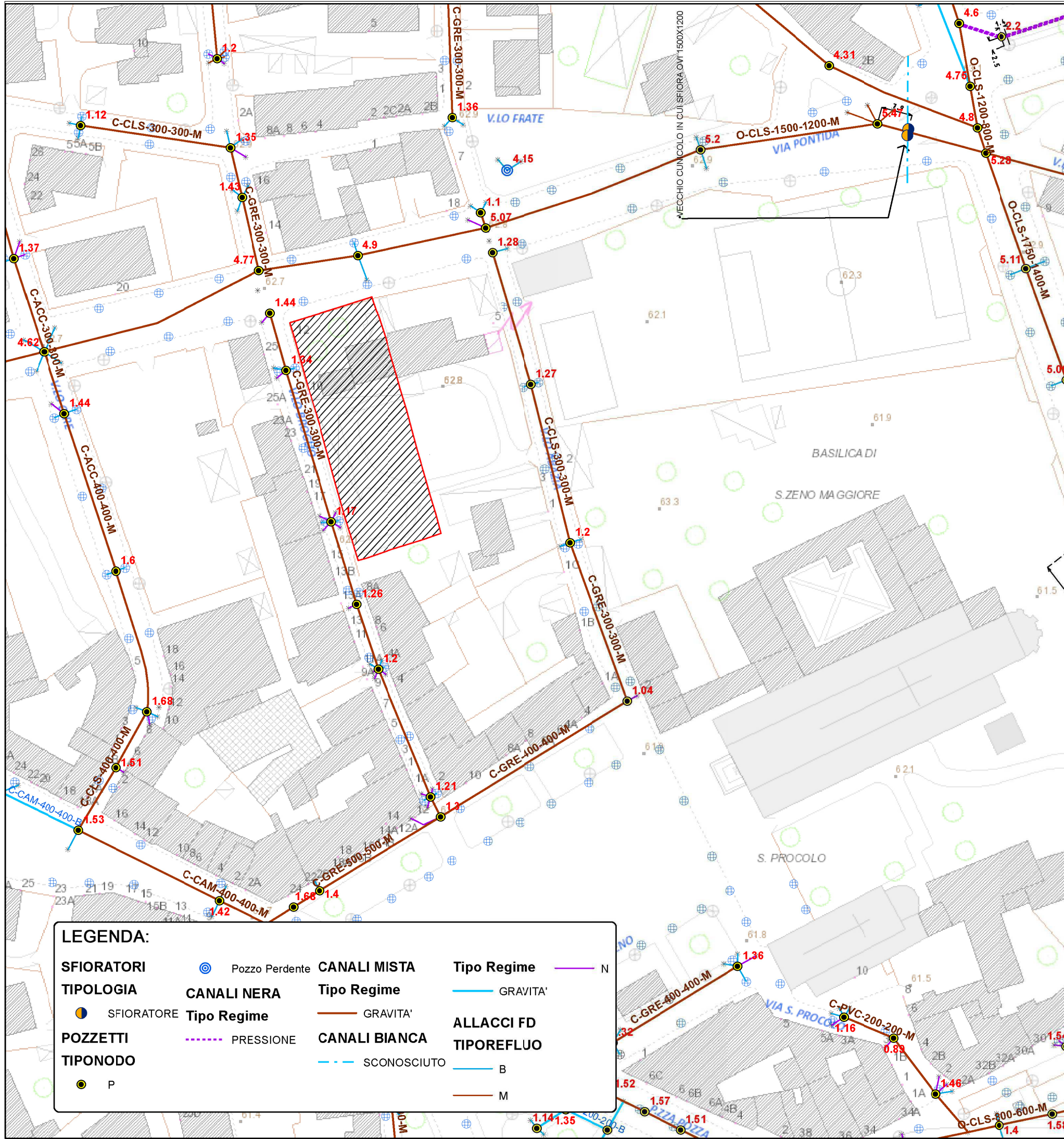
Schema rete fognatura
