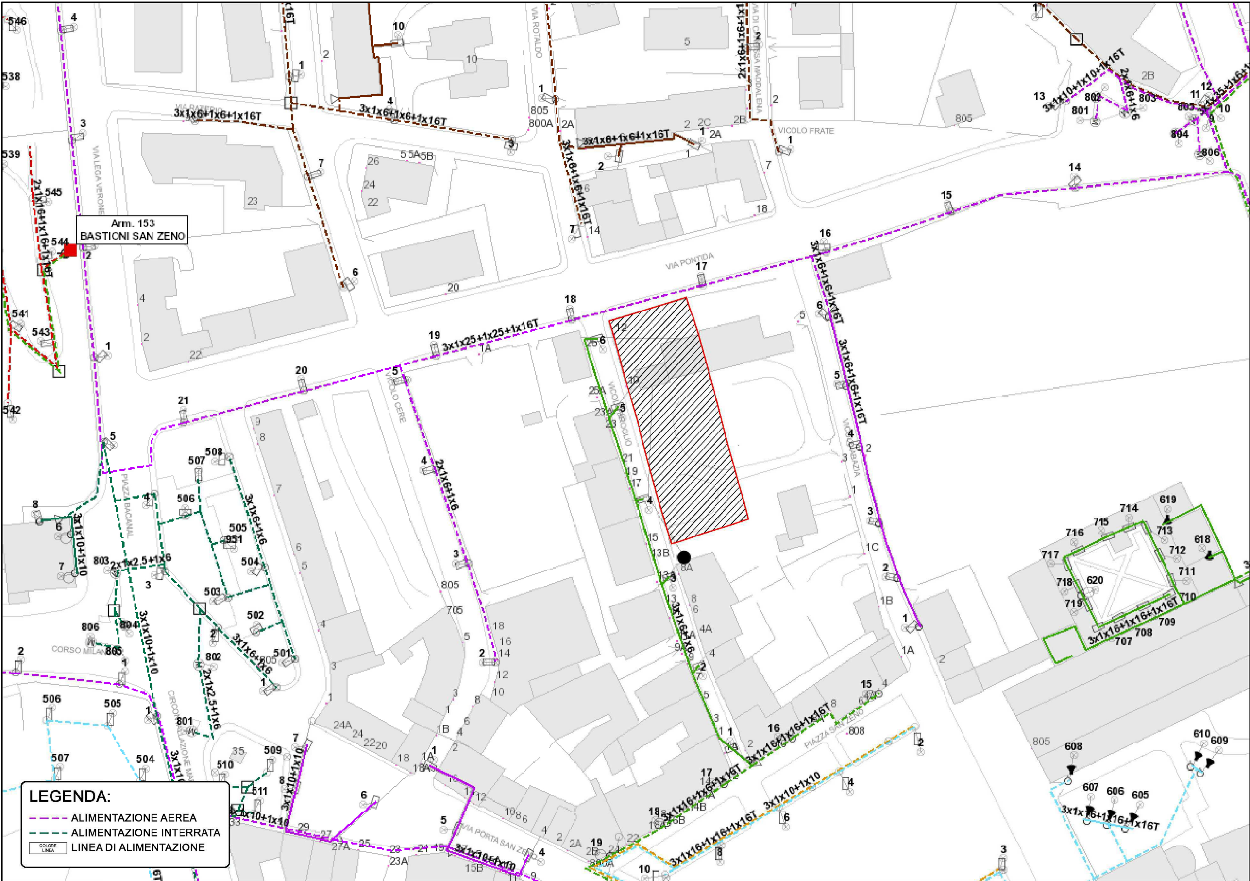
Schema rete illuminazione pubblica
