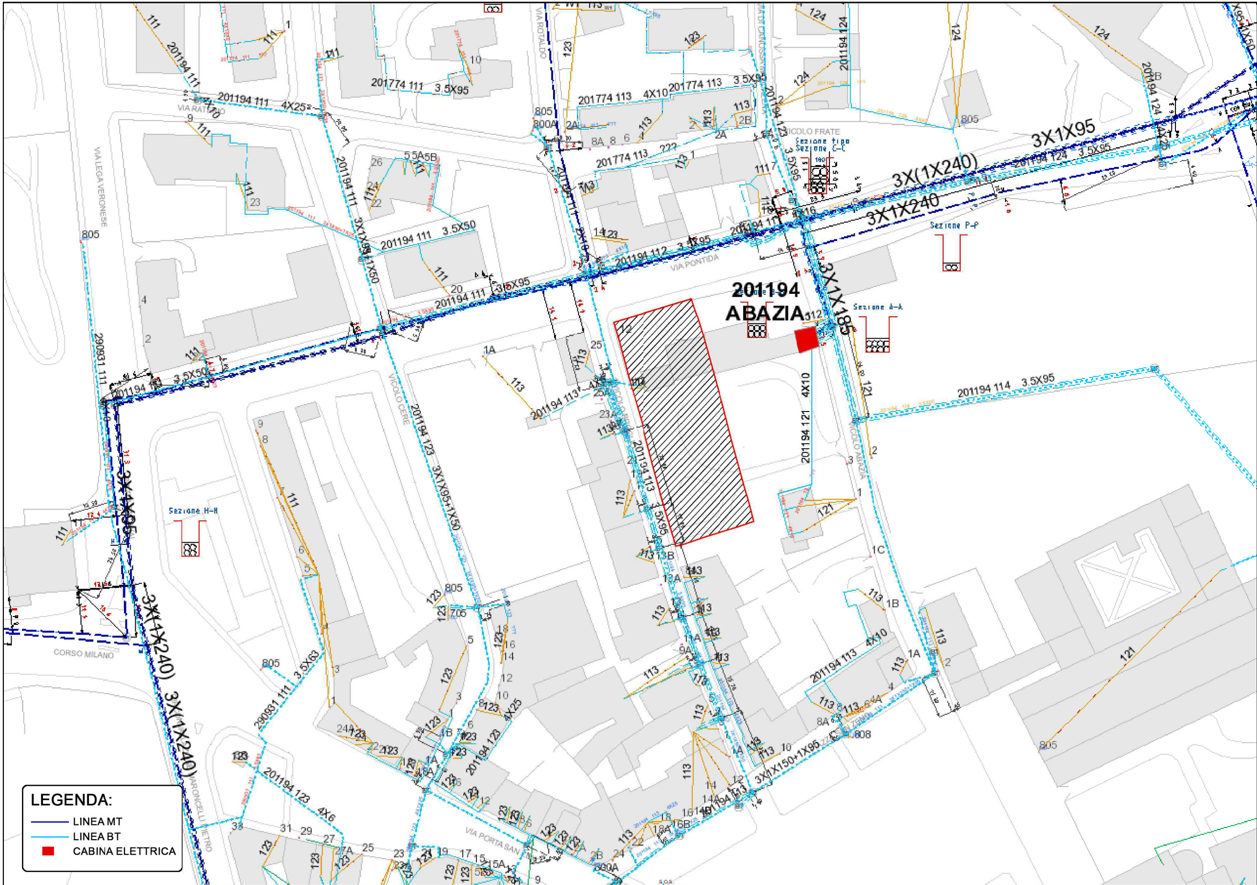
Schema rete elettrica
