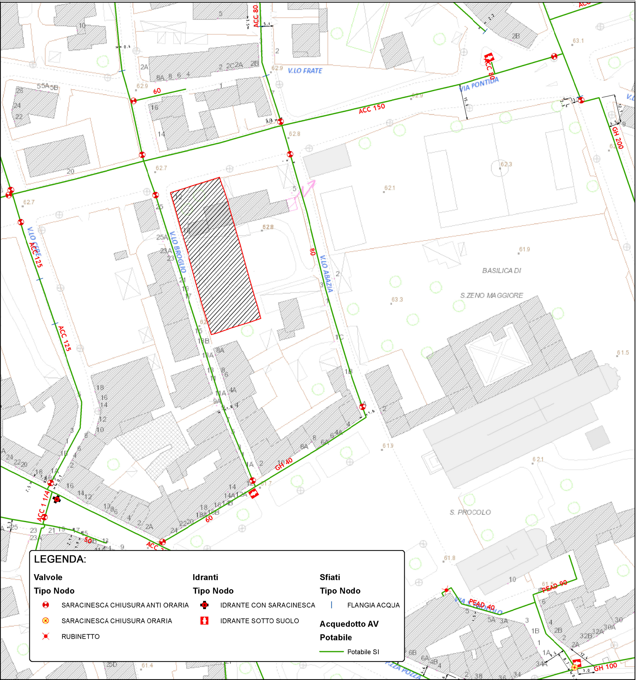
Schema rete acquedotto
